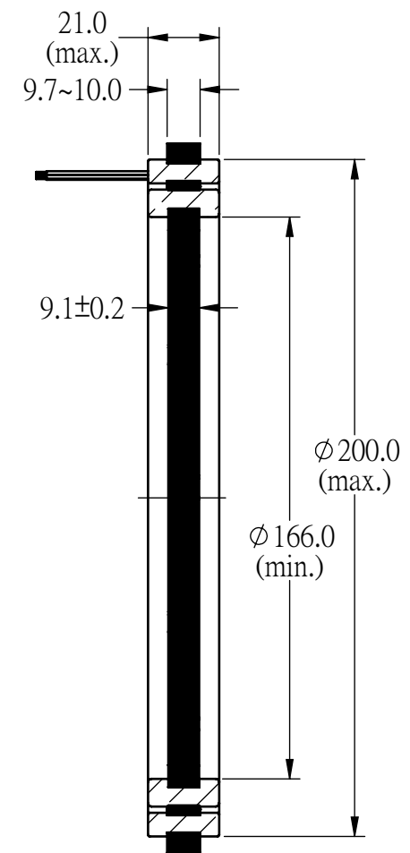
剖面圖 B-B
